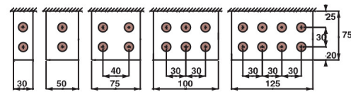
부스바 치수 (Terminal Dimesion)
