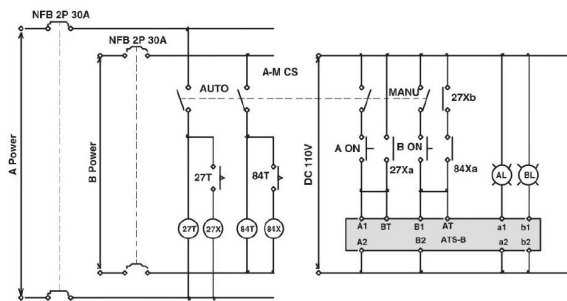
A,B Power : AC 220V
