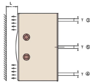
아크공간 (Arc space)
