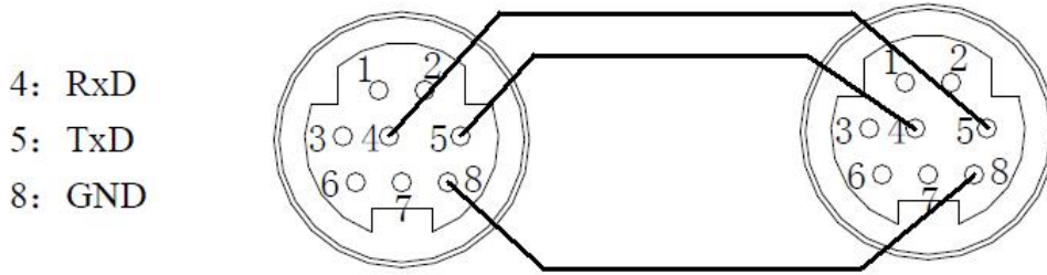
Mini Din 8 Pins port
